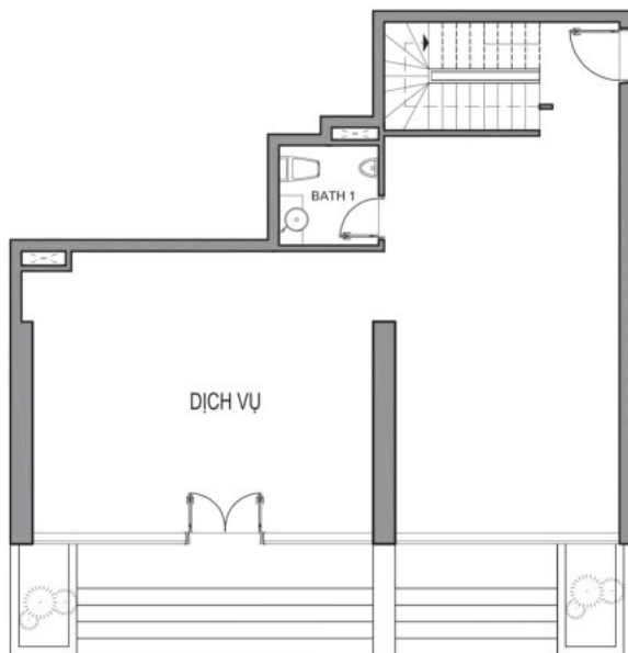
MẶT BẰNG TẦNG TRỆT
