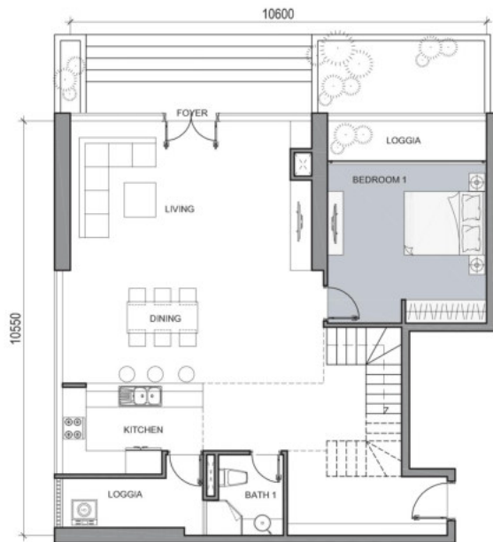
MẶT BẰNG TẦNG TRỆT
